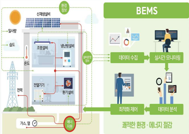
< 에너지고효율 신청사 개념도 >
